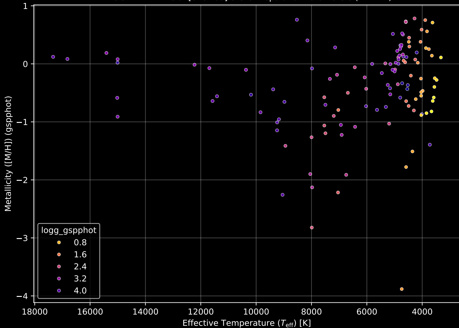
APOGEE DR17 Field: [018+00] Stellar Population Parameters (n= 124)
